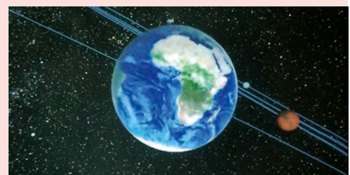
Mitaka プログラム:加藤恒彦 国立天文台4次元デジタル宇宙プロジェクト
